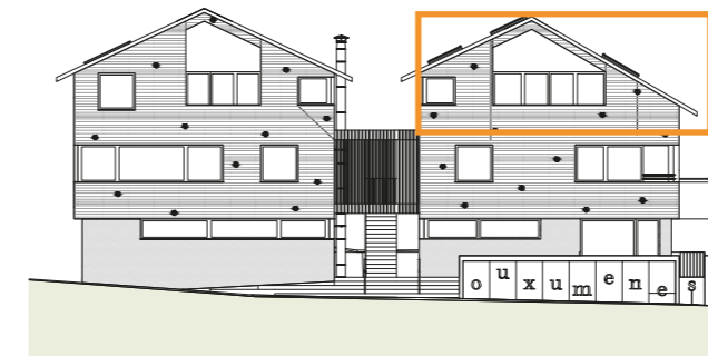
Dachgeschoß
